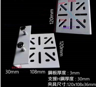
H-6 多孔 H 鋼夾
