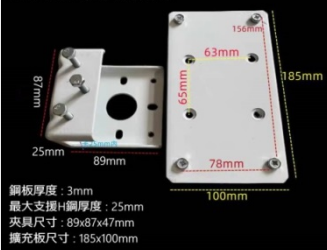
H-7 大型組合H鋼夾
